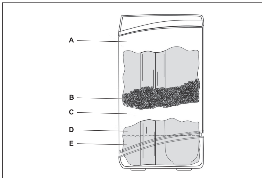
Abb. 2: Salzbrücke
