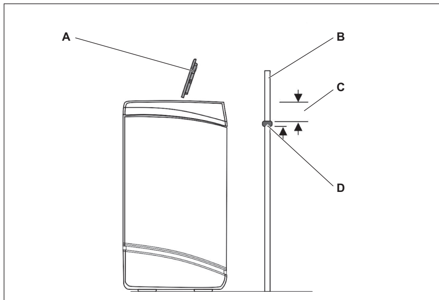
Abb. 3: Behälterhöhe markieren
