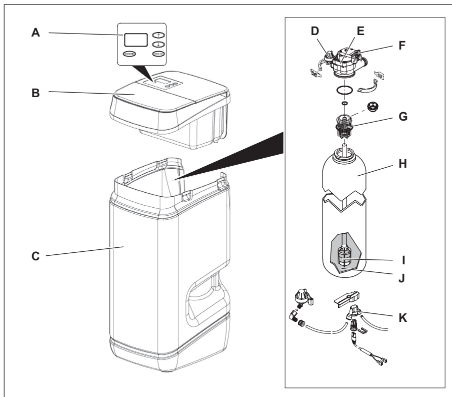
Abb. 1: Komponenten des Wasserenthärters
